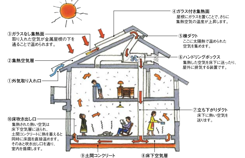
【パッシブソーラーの冬のしくみ】
